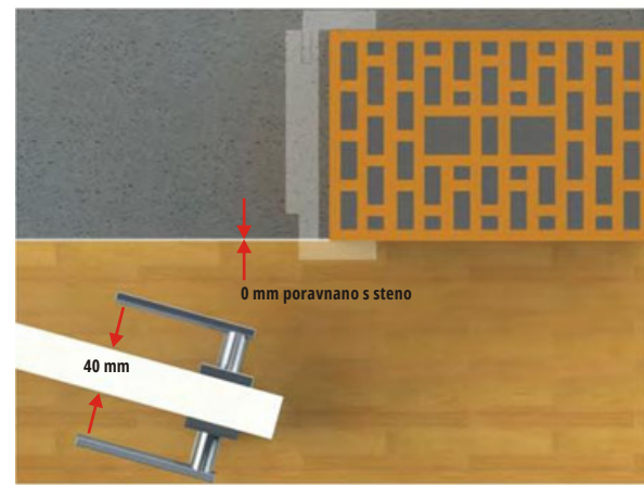
Podboj iz masivnega lesa s skritimi nasadili
