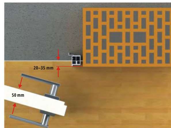
Aluminijast podboj s skritimi nasadili
