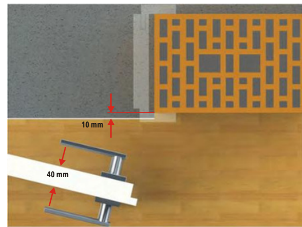
Podboj iz masivnega lesa z vidnimi nasadili
