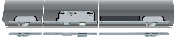
AUTOMATIK 6-Punktverriegelung mit Elektro-Motor
