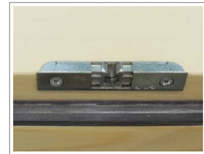
SCHNÄPPER Halter optional mit ETÖ (oben oder seitlich montiert)
